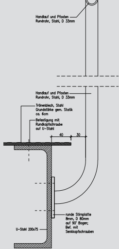
GELÄNDER ANSCHLUSS M 1:2.5
