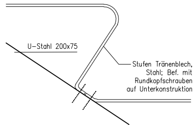
STUFENDETAIL M 1:2,5
