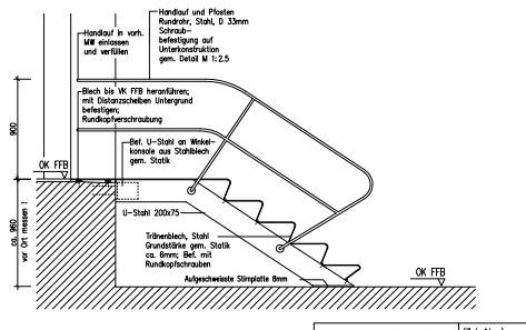
SCHNITT A-A M 1:25
